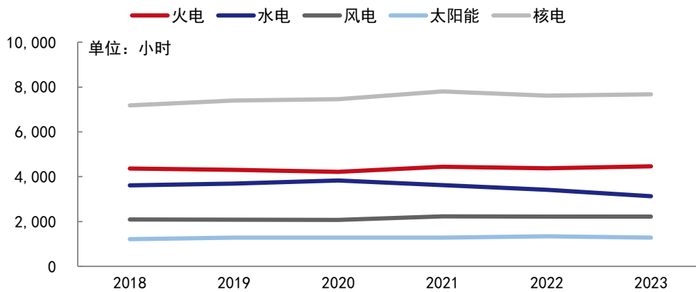
图4 我国不同电源类型机组发电利用小时数有所分化
