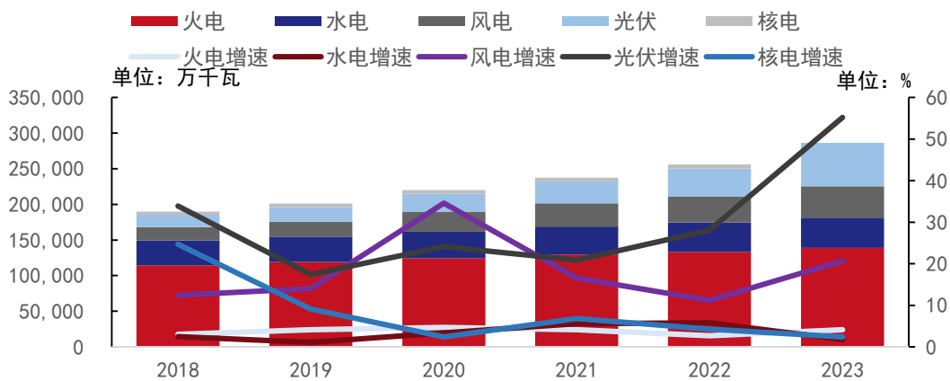
图2 我国火电和水电装机低速增长，风电、光伏装机保持相对较高增速
